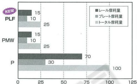
500時間運転後の摩耗量比較
